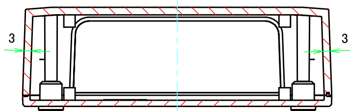
B-B ( 1 : 1.5 )
