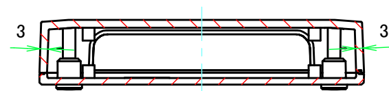
B-B (1:2)
