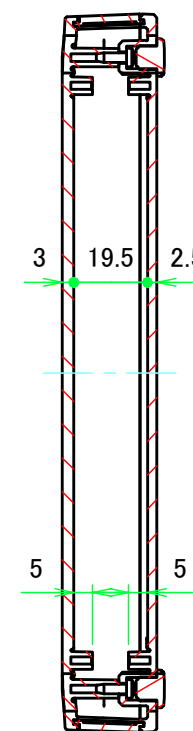
A-A (1:2)
