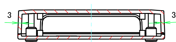
B-B (1:2)
