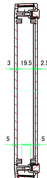
A-A (1:2)
