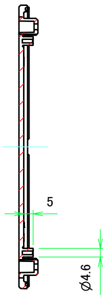
E-E ( 1 : 2 )
