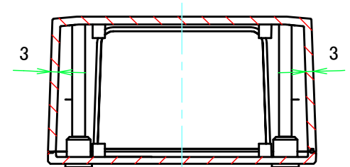
B-B ( 1 : 2 )
