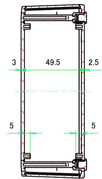
A-A ( 1 : 2 )
