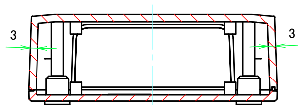
B-B ( 1 : 1.5 )
