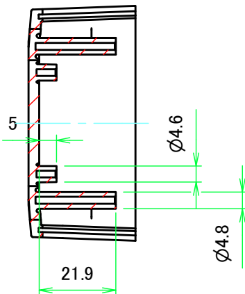
C-C ( 1 : 1.5 )
