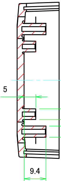
C-C ( 1 : 1 )
