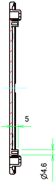
E-E ( 1 : 2 )
