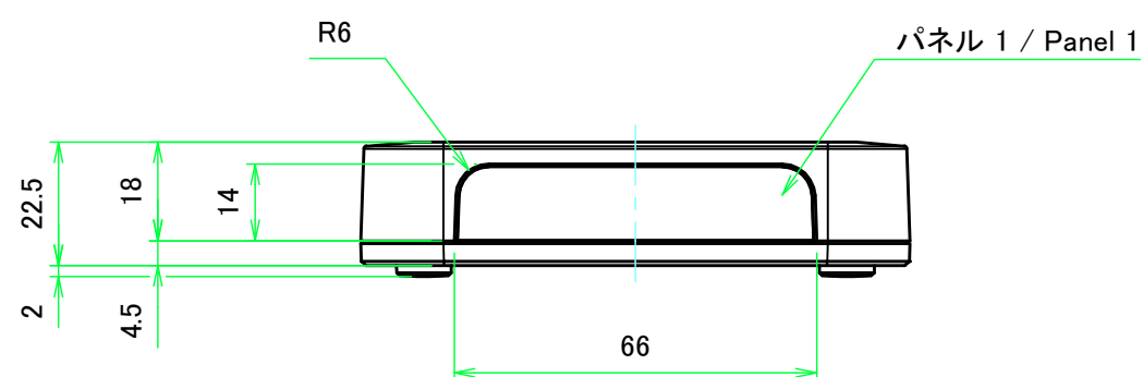
B-B ( 1 : 1.5 )
