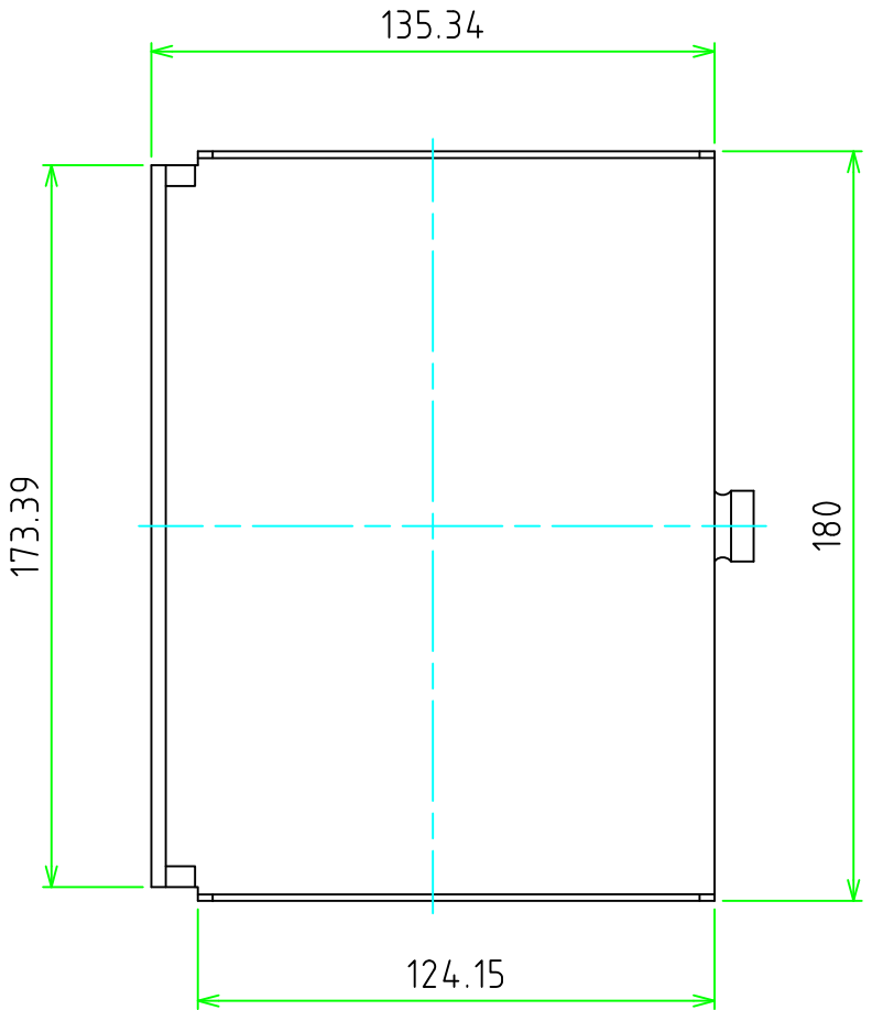
トップカバー (内視) Cover (Internal View)
