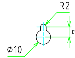
打抜き穴部詳細図 A A Detail : Hanging hole mark
