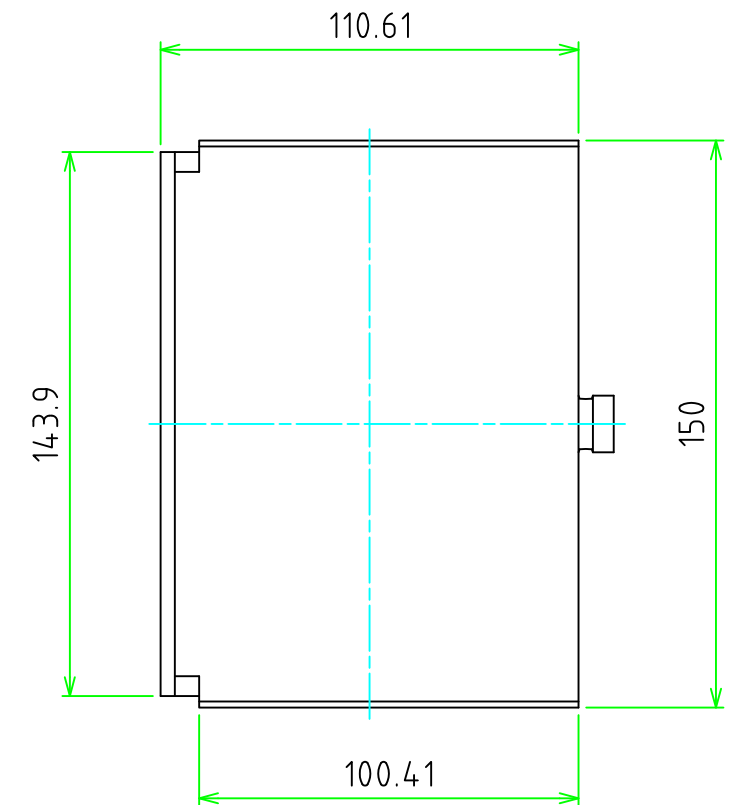
トップカバー (内視) Cover (Internal View)
