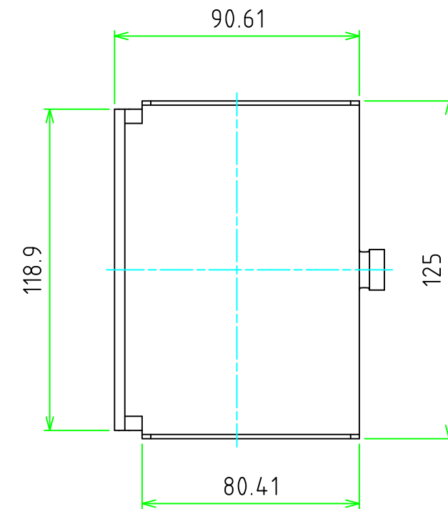
トップカバー (内視) Cover (Internal View)
