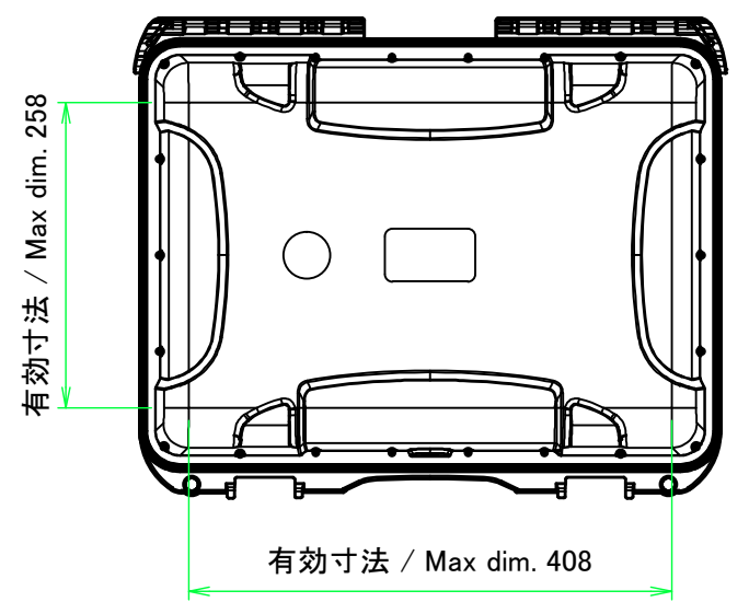
ベース 内視 / Base Internal view
