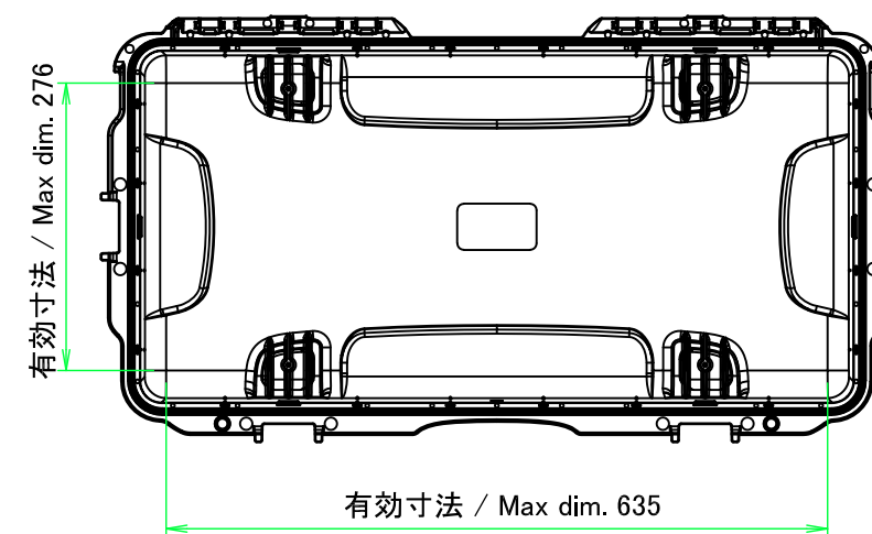
ベース 内視 / Base Internal view
