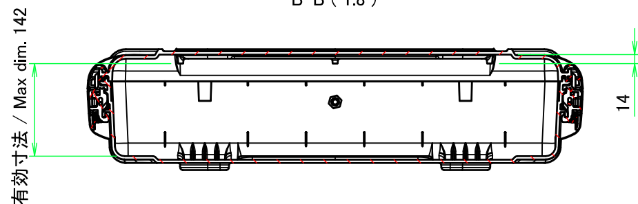
B-B ( 1:8 )
