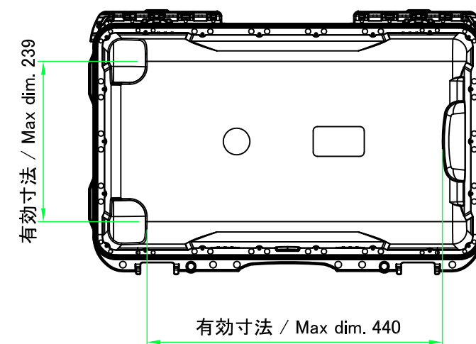
ベース 内視 / Base Internal view
