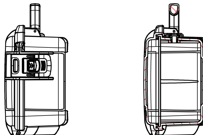
A-A (1:4)
