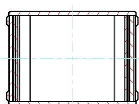
C-C (1:2)
