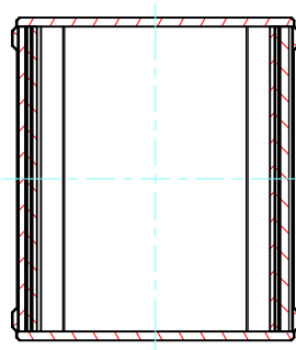
C-C (1:2)
