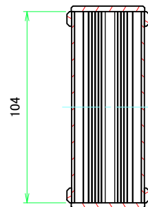
B-B (1:2)
