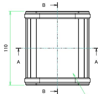
本体フレーム1 Frame 1
