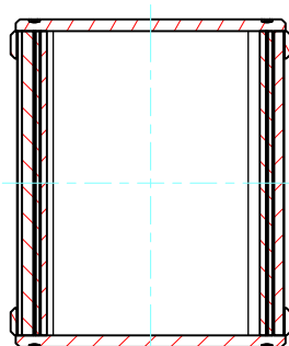
D-D (1:1.5)
