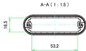
A-A (1:1.5)
