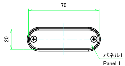
A-A (1:1.5)
