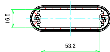
A-A (1:1.5)
