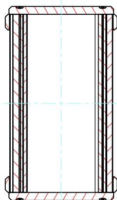
D-D (1:1)
