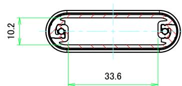
A-A (1:1)
