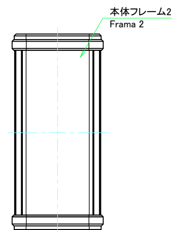
D-D (1:1.5)
