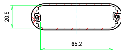
A-A (1:1.5)
