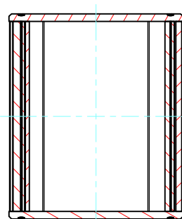
D-D (1:1.5)
