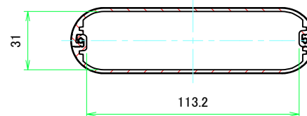
A-A (1:2)
