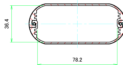
A-A (1:1.5)
