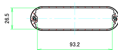
A-A (1:2)
