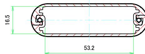
A-A (1:1)
