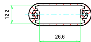
A-A (1:1)
