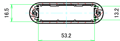
A-A (1:1.5)
