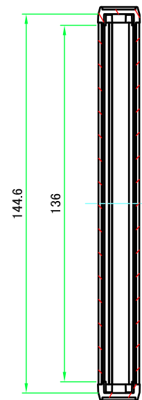
B-B (1:2)
