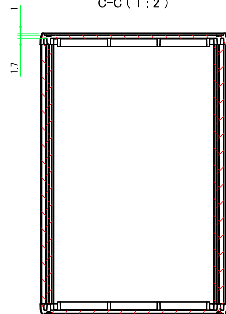
C-C (1:2)
