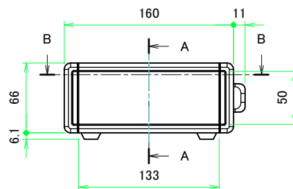
フロントフレーム2 / Front frame2
