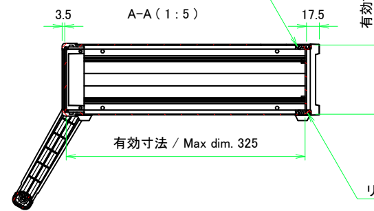
リアフレーム1 / Rear frame1
