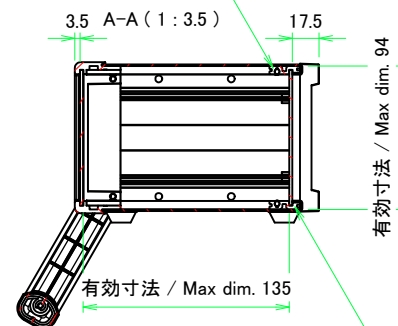
リアフレーム1 / Rear frame1
