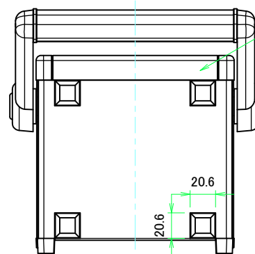
フロントフレーム2 / Front frame2
