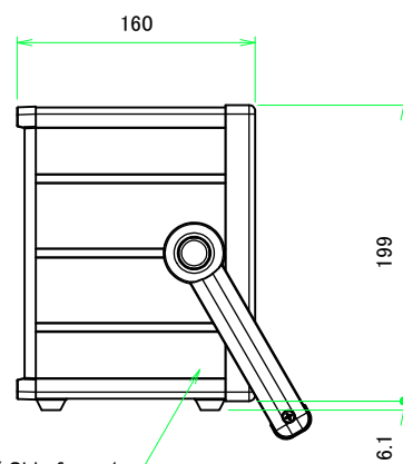
サイドフレーム1 / Side frame1
