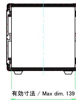
リアフレーム2 / Rear frame2
