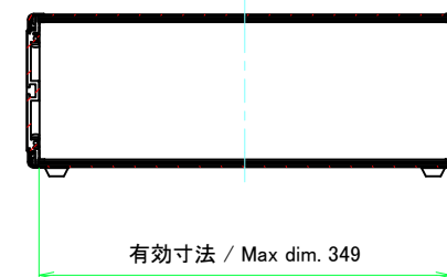
リアフレーム2 / Rear frame2
