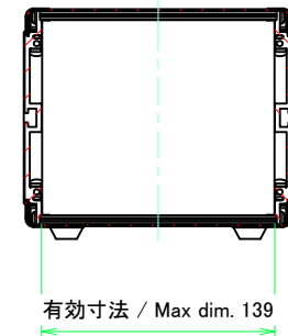
C-C (1:3.5)
