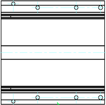
サイドフレーム2 / Side frame2
