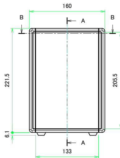
フロントフレーム1 / Front frame1
