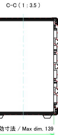
リアフレーム2 / Rear frame2
