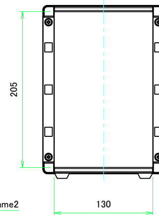
リアフレーム2 / Rear frame2
