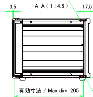
リアフレーム1 / Rear frame1
