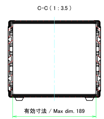
リアフレーム2 / Rear frame2
