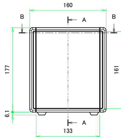
フロントフレーム1 / Front frame1
