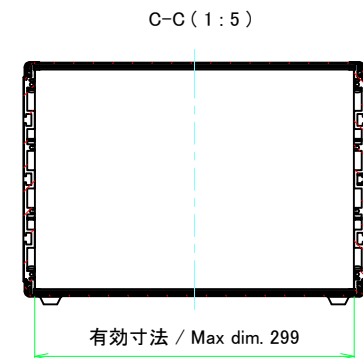
リアフレーム2 / Rear frame2
