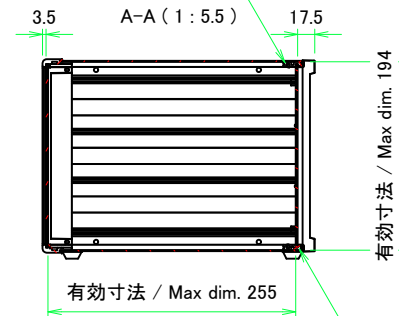
フロントフレーム1 / Front frame1
