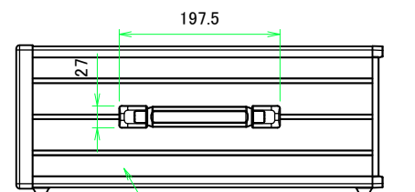
フロントフレーム1 / Front frame1
