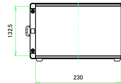
サイドフレーム2 / Side frame2
