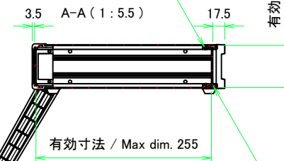
リアフレーム1 / Rear frame1
