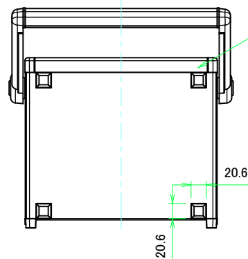
フロントフレーム2 / Front frame2
