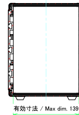
C-C (1:3.5)
